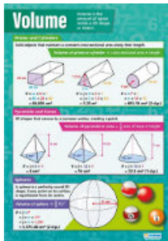
Volume
